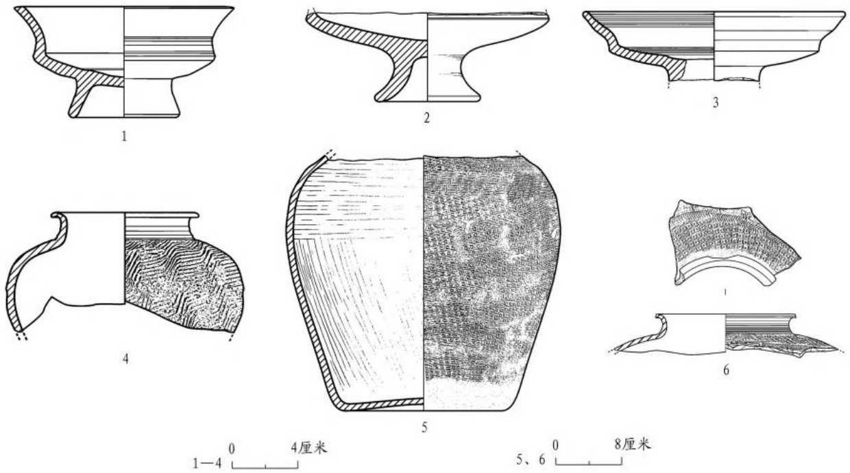
图一四// 原始瓷、印纹硬陶器
