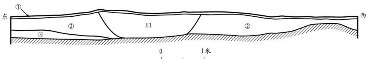
图四// T0202南壁剖面图
