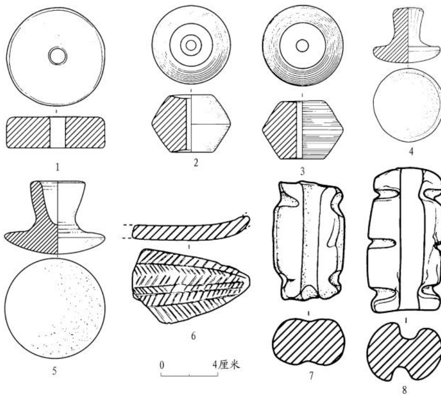
图一三// 陶制生产工具
