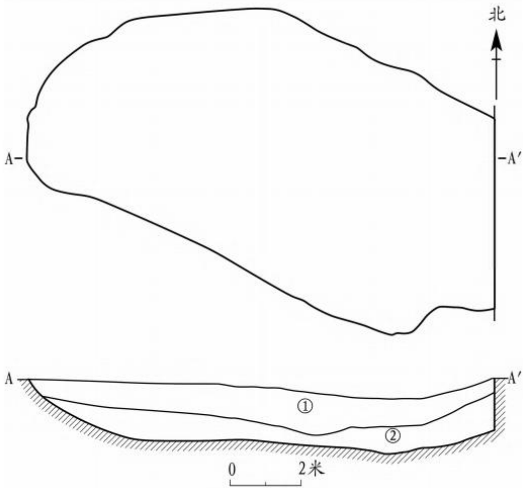
图五// H5平、剖面图
