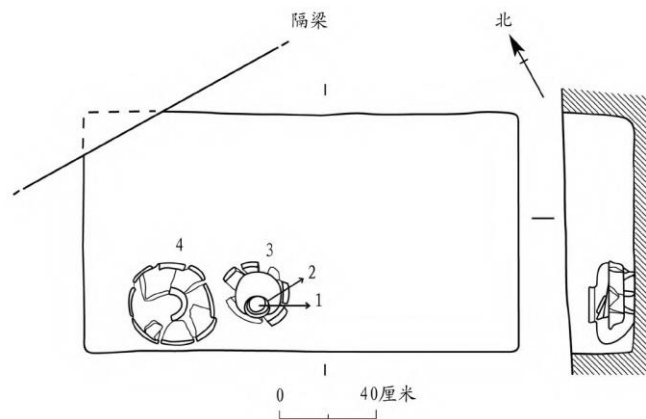
图九//M4 平、剖面图
