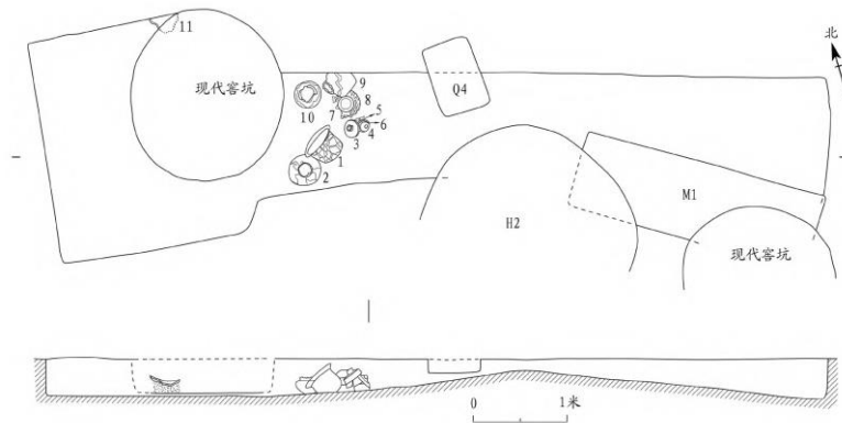
图八//M3 平、剖面图
