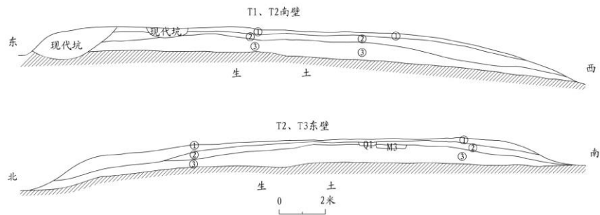
图三//D2 地层堆积剖面图
