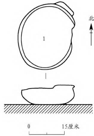
图一三//Q3 平、剖面图
