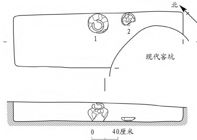
图五//M1 平、剖面图
