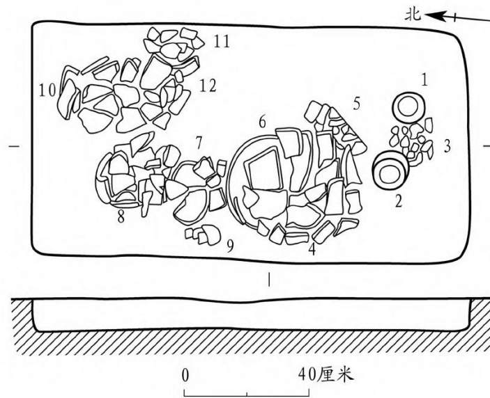
图一七//Q6 平、剖面图
