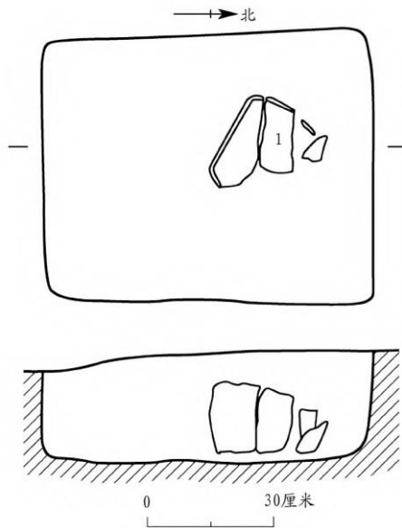
图一四//Q4 平、剖面图
