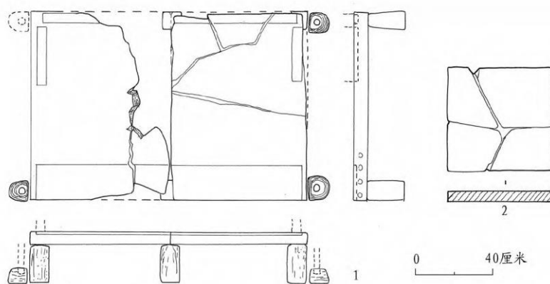
图一〇//M41 出土石器
