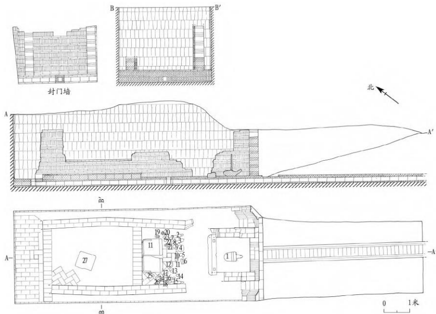
图五//M41 平、剖面图
