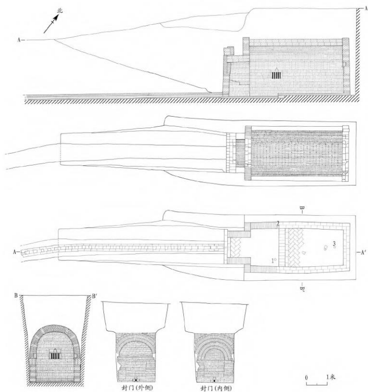
图三//西善桥刘家村 M9 平、剖面图
