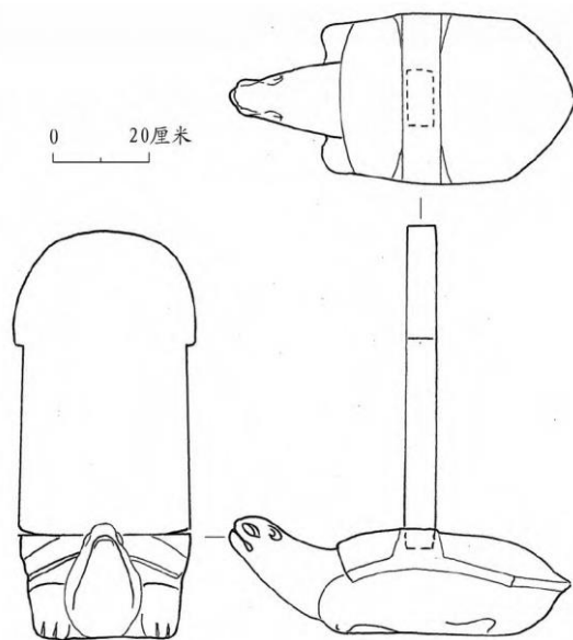
图八//M41 出土石龟趺墓志 (M41 : 1)
