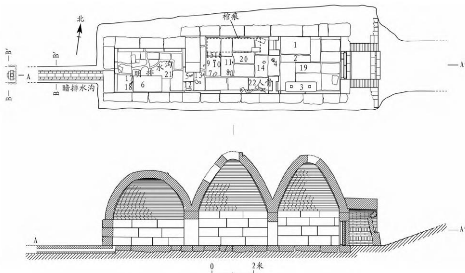
图二//M1 平、剖面图
