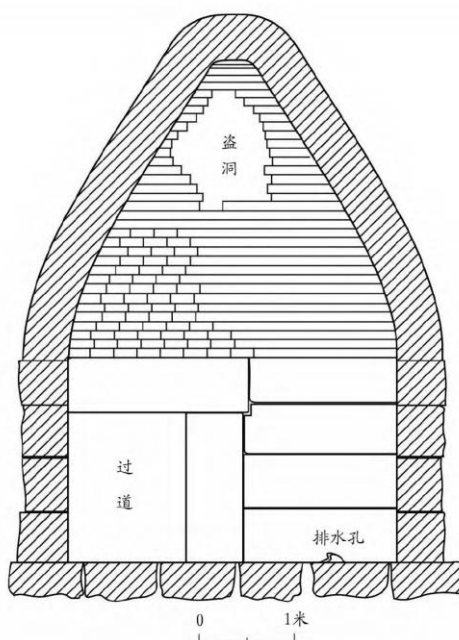
图五//中室西壁剖面图
