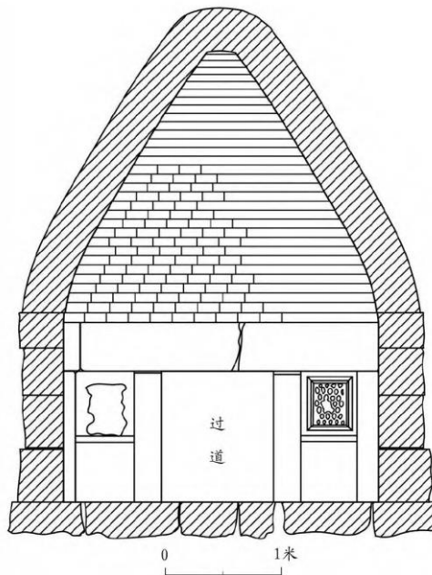
图四//前室西壁剖面图
