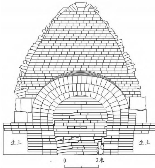
图三//封门墙、甬道正视图
