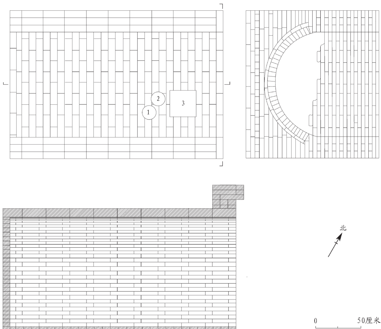
图二// 吴山岭明墓平、剖面图
